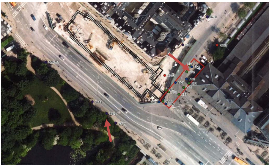
Figur 2. Angivelse af brønd, hvor rørledningen indføres i vandløbet (øverste pil), stemmeværket og re-infiltrationsbrønde (nederste pil, start og slut).
