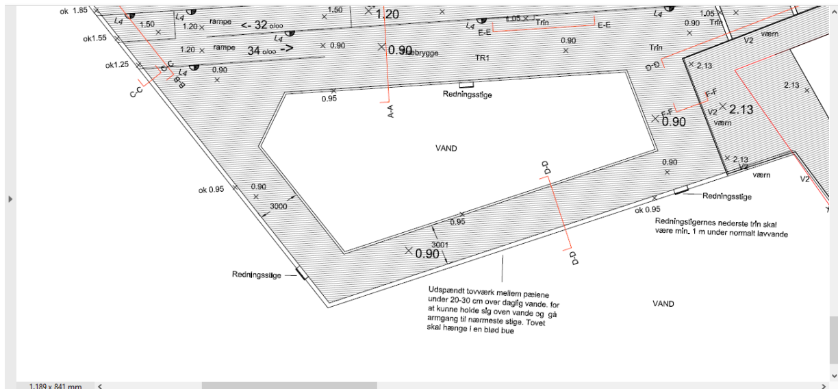
Skitse af Teglholm Brygge 1:200
