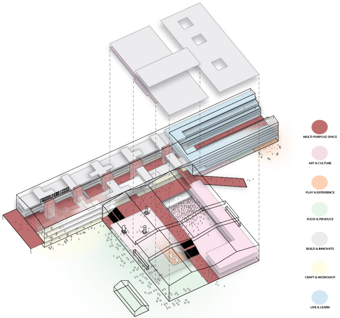
Isometri af Tunnelfabrikken
